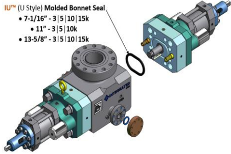
7-1/16" IU™ (U Style) Bonnet Door Seal
