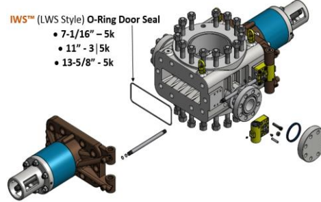
7-1/16" IWS™ (LWS Style) O-Ring Door Seal
